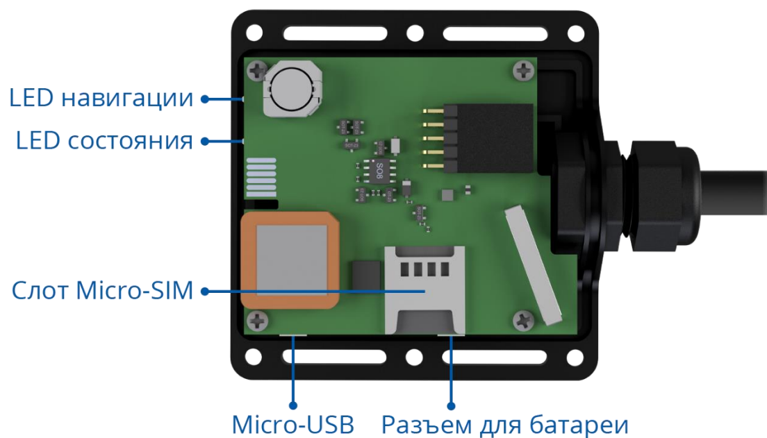
Вид снизу (без крышки)
