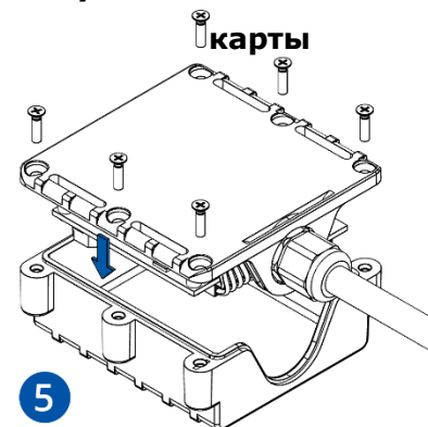
5 Рисунок 8 Прикрепление крышки
